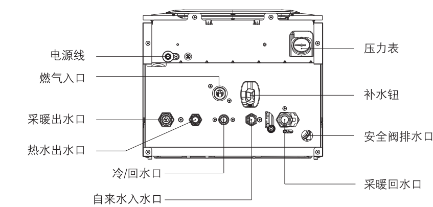
壁挂炉底部结构
